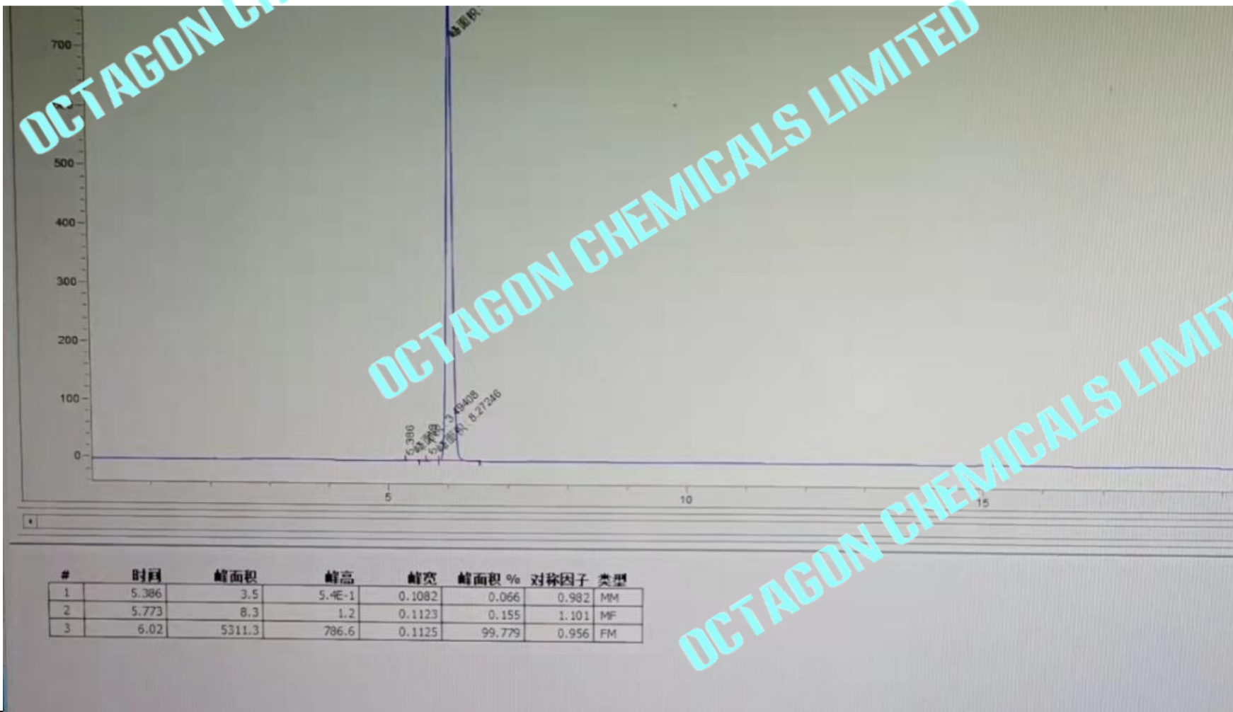
Alpha-estradiol Cas 57-91-0 HPLC Spectrum
