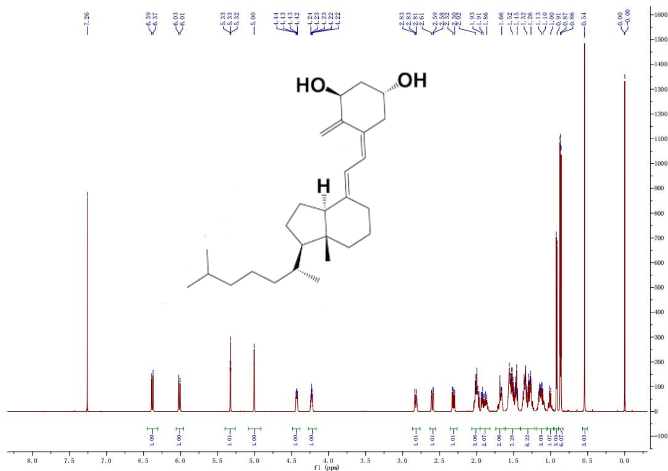
Alfacalcidol Cas 41294-56-8 1HNMR Spectrum
