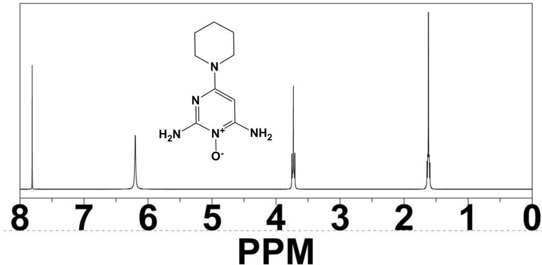
Minoxidil 38304-91-5 1 HNMR Spectrum
