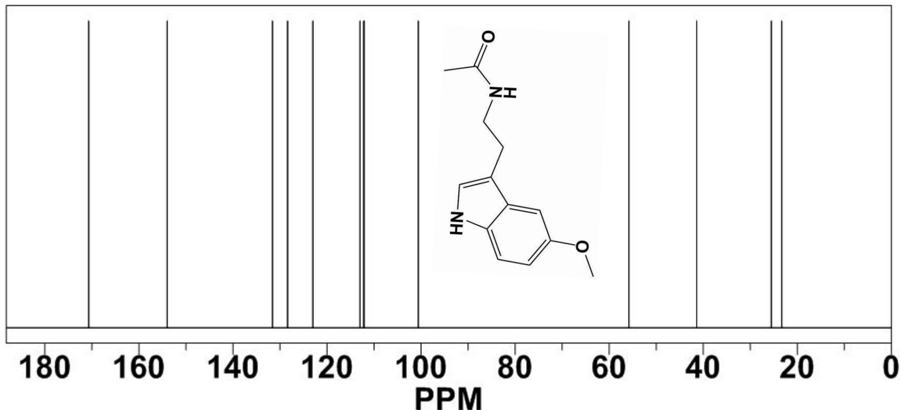
Melatonin 73-31-4 13 CNMR Spectrum
