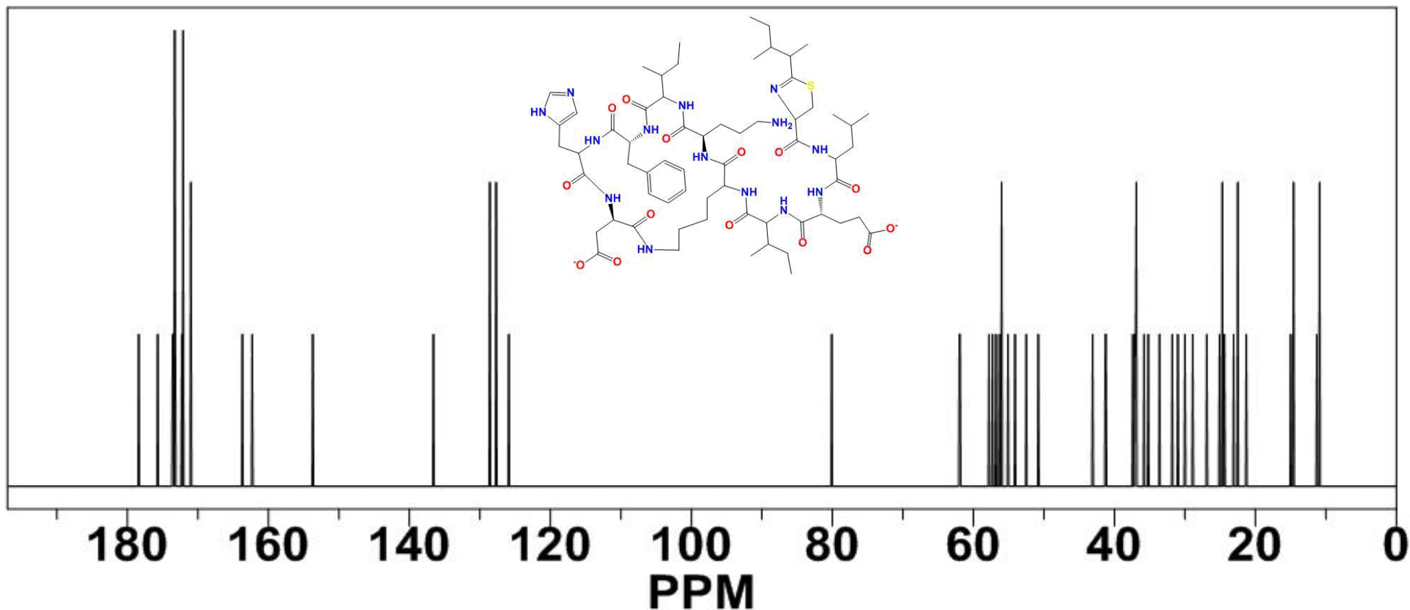
Bacitracin 1405-87-4 13 CNMR Spectrum
